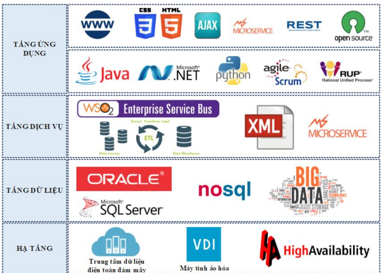
Sơ đồ 7: Các tầng kiến trúc công nghệ
