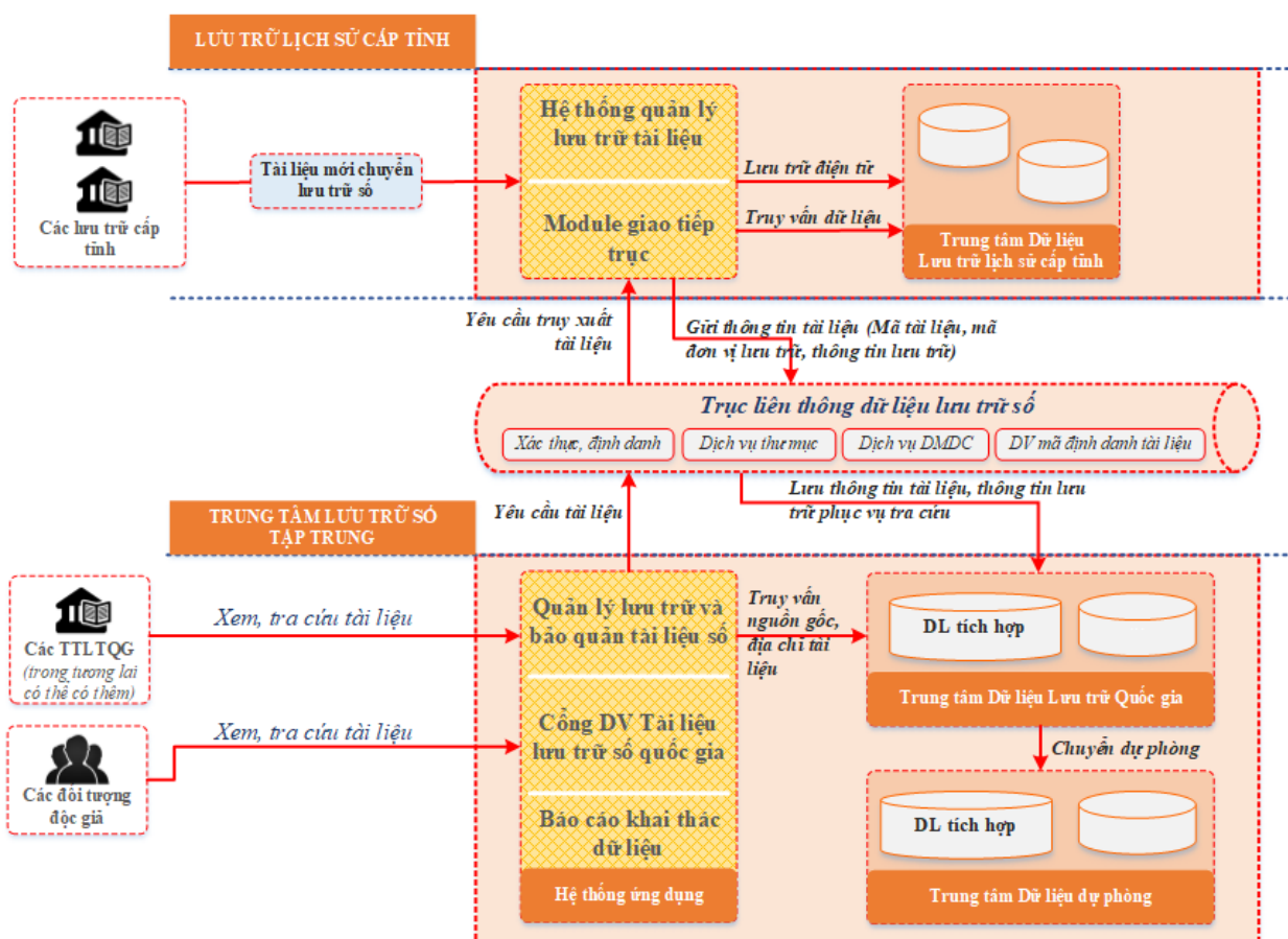
Sơ đồ 4: Mô hình nguyên lý tạo lập liên kết và trao đổi dữ liệu giữa Lưu trữ lịch sử cấp tỉnh, Lưu trữ chuyên ngành và Trung tâm Dữ liệu Lưu trữ số tập trung
